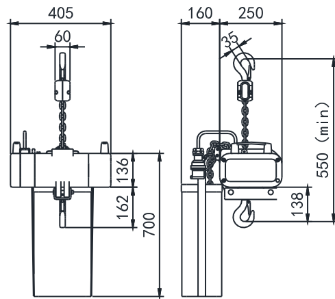
单刹车 Single brake
