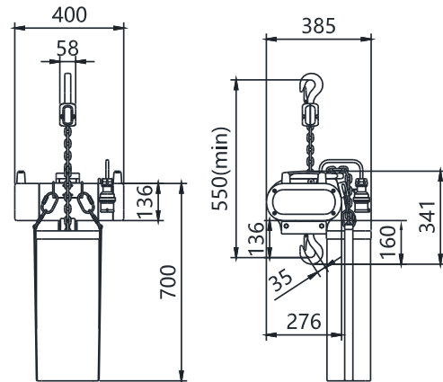
单刹车 Single brake
