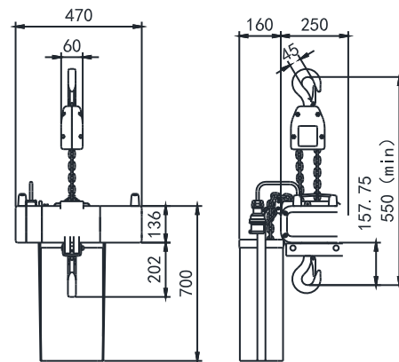
双刹车 Double brakes
