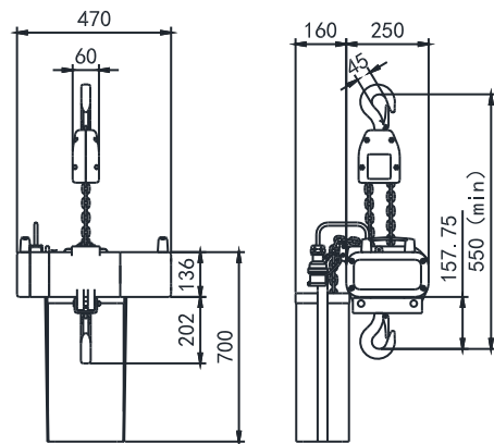
双刹车 Double brakes
